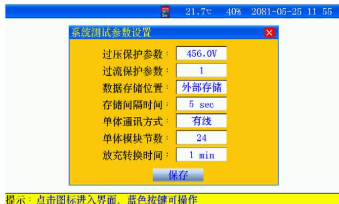
图 3.16 放充转换时间设置界面
