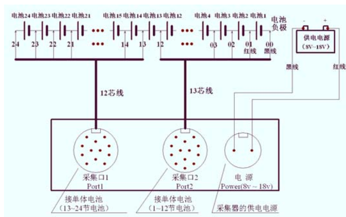
图 2.4.4 24 节 2V 电池与 1 个单体模块连接图
