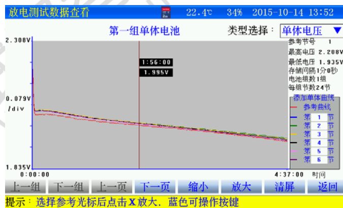
图 3.7.4-1 单体电压曲线界面
