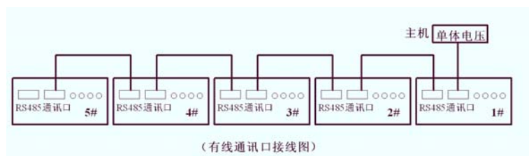
图 2.4.4-4 有线通讯口接线图
