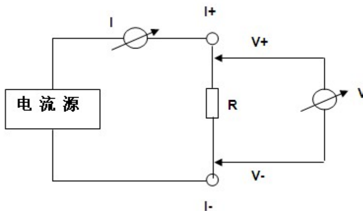
图 1 测试原理图
